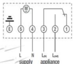
Wiring diagram - Volt Free Switching
